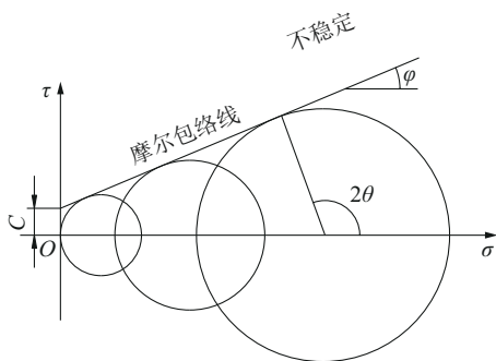
图4 岩石破坏摩尔包络线图
