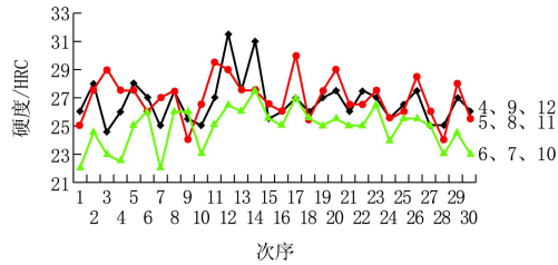
图 11 1 号配方 8 mm 高度胎体第 1 次磨 1 mm 后硬度曲线
