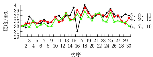
图 23 2 号配方 6 mm 高度胎体第 5 次磨 1 mm 后硬度曲线
