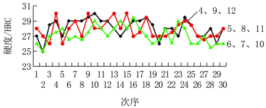
图 15 1 号配方 8 mm 高度胎体第 5 次磨 1 mm 后硬度曲线
