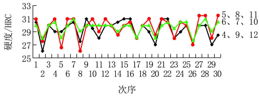
图 17 1 号配方 8 mm 高度胎体第 7 次磨 1 mm 后硬度曲线
