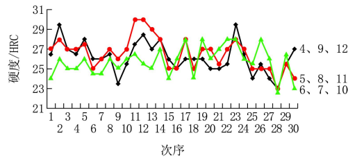
图 13 1 号配方 8 mm 高度胎体第 3 次磨 1 mm 后硬度曲线
